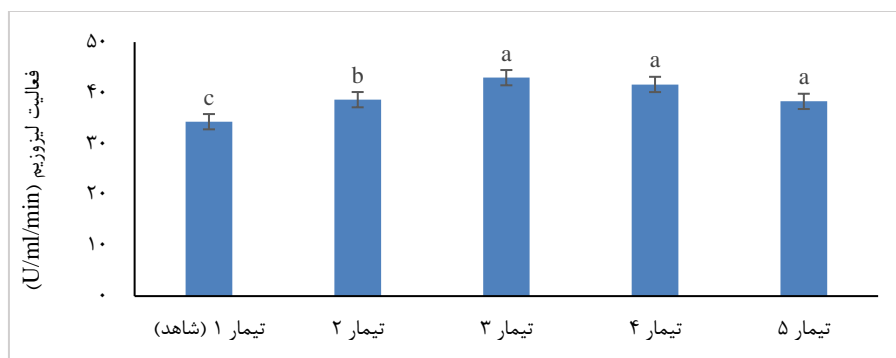
شکل ۱- میانگین فعالیت لیروزیم (U/ml/min) بچه ماهیان قزل آلابی رنگین کمان در رویارویی با استامینوفن در پایان دوره آزمایش. حروف لاتین غیر همنام تفاوت معنادار را نشان می‌دهد ( p < 0.05 )
