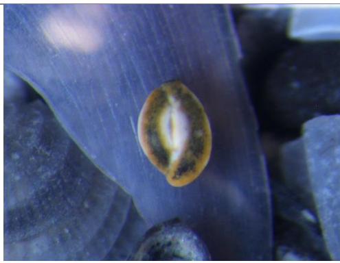
(۳-۲): Spiroloculina sp.
