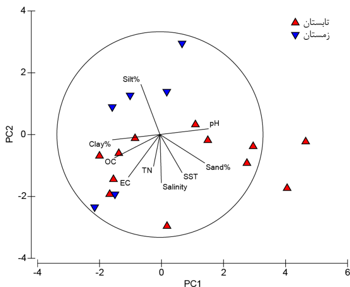
شکل ۴. آزمون مؤلفه‌های اصلی داده‌های محیطی در جنگل حرای خور خوران (SST=دمای سطحی آب؛ OC=کربن آلی؛ TN=نیترژن کل؛ EC=هدایت الکتریکی؛ Sand%=درصد شن؛ Silt%=درصد لای؛ Clay%=درصد رس؛ Salinity=شوری؛ pH=اسیدیته)
