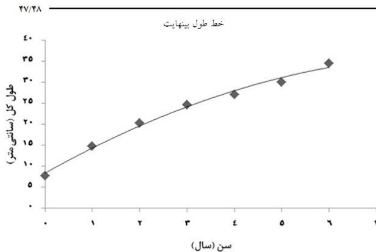
شکل ۳ رابطه طول کل - سن لای ماهی صید شده در تالاب انزلی.
