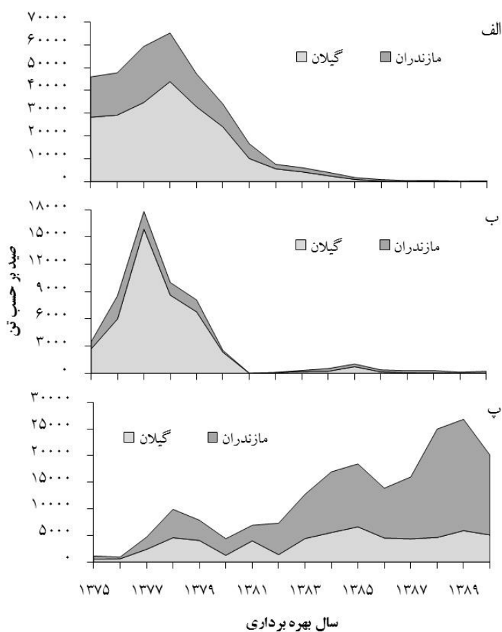
شکل ۴ الف - میزان صید ماهی کیلکای آنچوی، ب - کیلکای چشم‌درشت و پ - کیلکای معمولی، در سواحل ایرانی دریای خزر در دو منطقه مازندران و گیلان طی سال‌های ۱۳۷۵ تا ۱۳۹۰.
