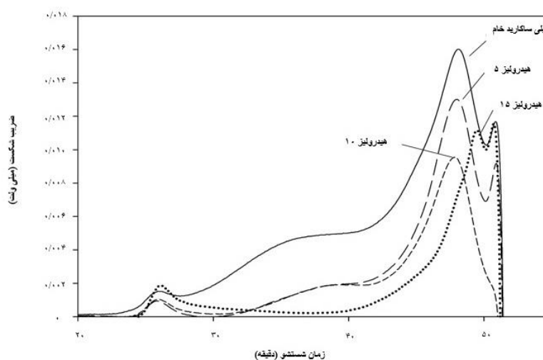
شکل ۱- نمودار شویش پلی ساکاریدهای خام و هیدرولیزات A. ficuloides بر روی ستون کروماتوگرافی BioSep-SEC-s2000
