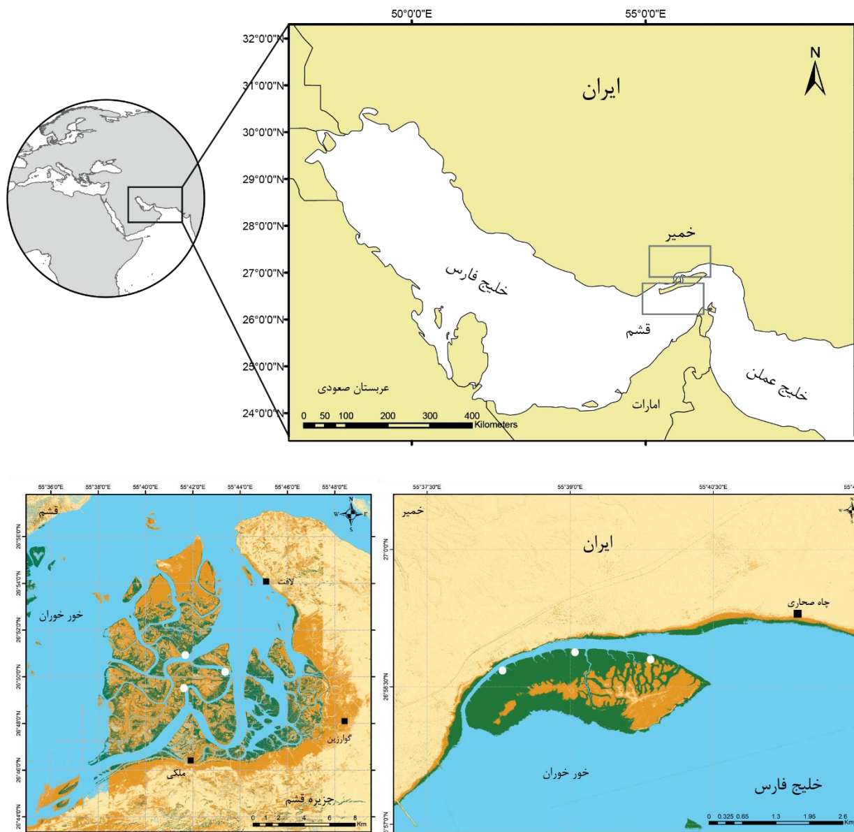
شکل ۱. منطقه‌های اصلی نمونه‌برداری در خلیج فارس و دریای عمان
