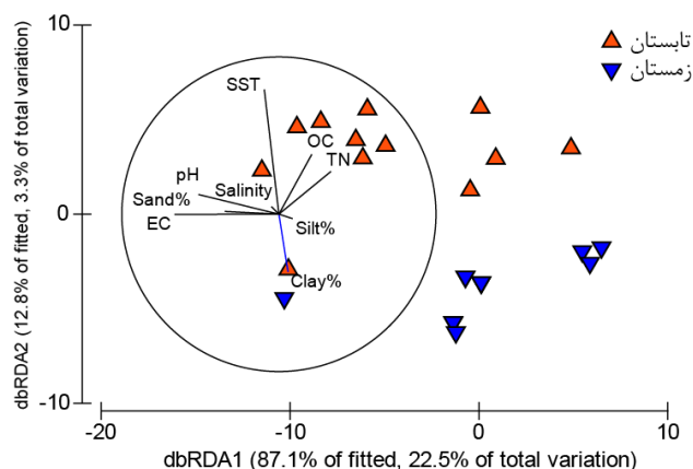
شکل ۵. آزمون افزونگی داده‌های محیطی در دو فصل تابستان و زمستان در جنگل حرای خور خوران؛ (SST= دمای سطحی آب؛ OC= کربن آلی؛ TN= نیتروژن کل؛ EC= هدایت الکتریکی؛ Sand%= درصد شن؛ Silt%= درصد لای؛ Clay%= درصد رس؛ Salinity= شوری؛ pH= اسیدیته)
