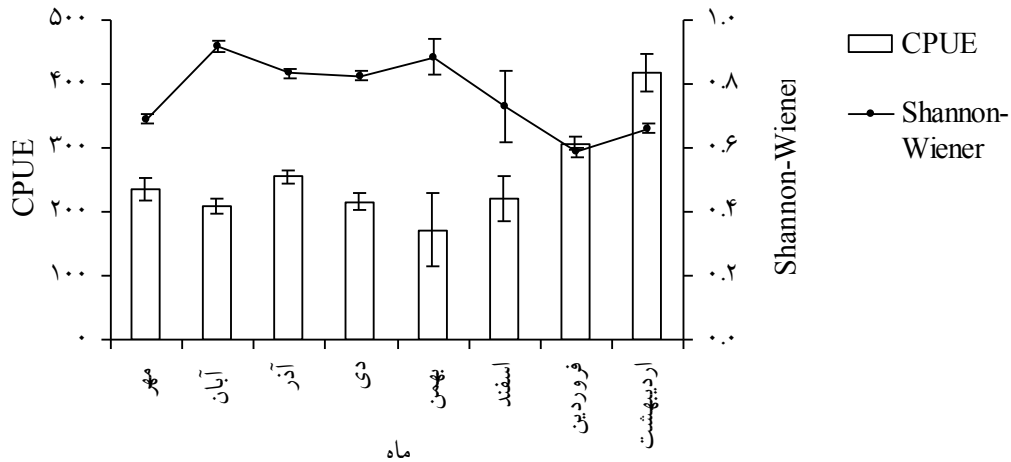
شکل ۲ میانگین (خطای معیاری ±) CPUE (صید در هر بار پره‌کشی بر حسب کیلوگرم) و شاخص تنوع شانون-وینر ماهیان استخوانی در پره‌های صیادی در ماه‌های مختلف.
