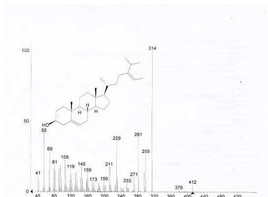
شکل ۱. کروماتوگرام و طیف کروماتوگرافی حاصل از فرکشن شماره ۱۸ (ان هگزان - اتیل استات ۱۰: ۴۰)، حاوی ترکیب Stigmasta-5,24(28)-dien-3-ol,(3 \beta -24Z)
