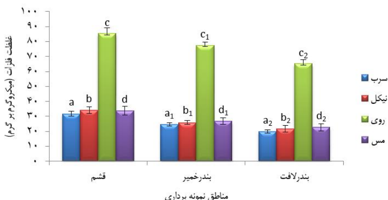
شکل ۲. مقایسه عناصر سرب، نیکل، روی و مس در در رسوبات، سه منطقه قشم، بندرخمیر و بندرلافت. حروف نامشابه در هر ستون بیانگر وجود اختلاف معنی دار ( p < 0.05 ) است.
