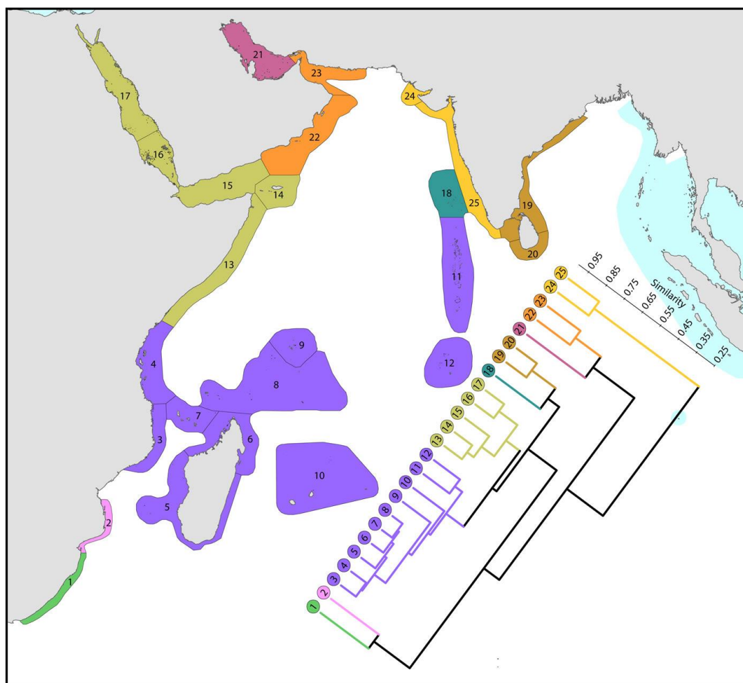
شکل ۱- کلاдоگرام شباهت نواحی اکولوژیک خلیج فارس و دریاهای همسایه بر اساس اشتراک گونه‌های آبسنگ مرجانی (برگرفته از Veron, 2016)
