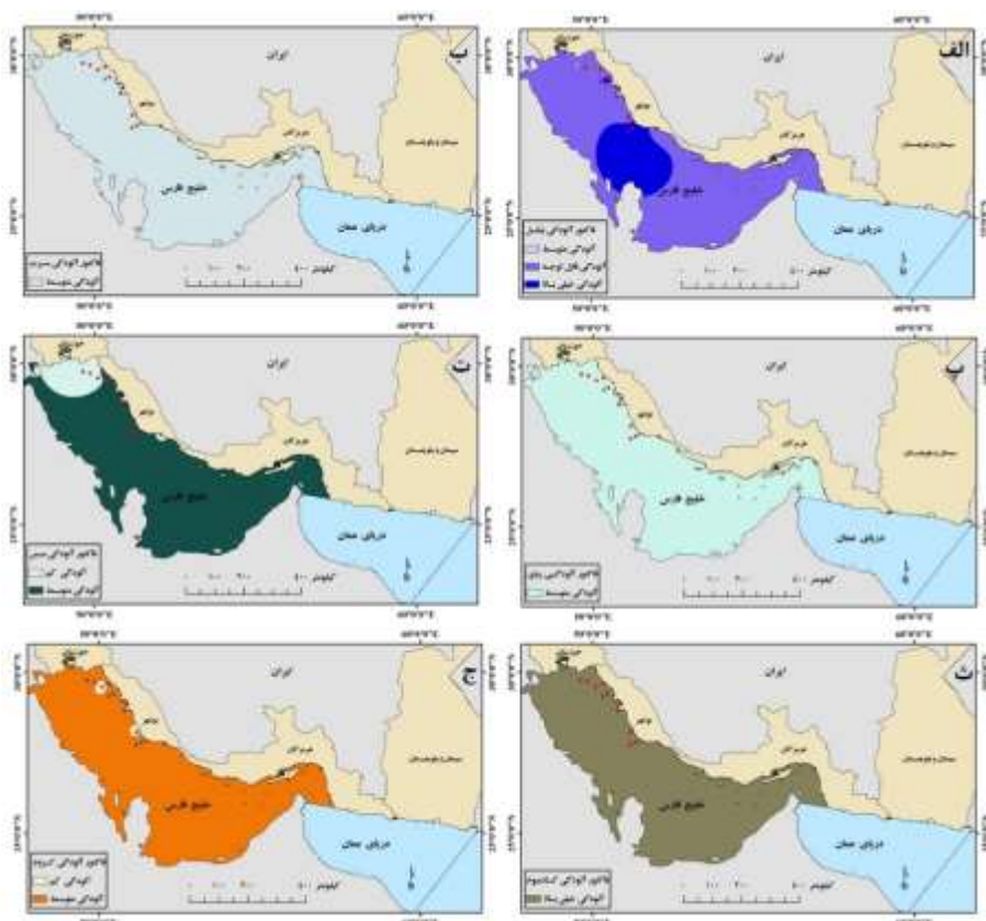
شکل ۶. الگوی پراکنش مکانی فاکتور آلودگی (CF فلزات سنگین الف) نیکل، ب) سرب، پ) روی، ت) مس، ث) کادمیوم و ج) کروم، خلیج فارس، سال ۱۳۹۹ (توجه شود که تنها الگوی پراکنش مکانی در اطراف ایستگاه‌های نمونه‌برداری مد نظر می‌باشد).
